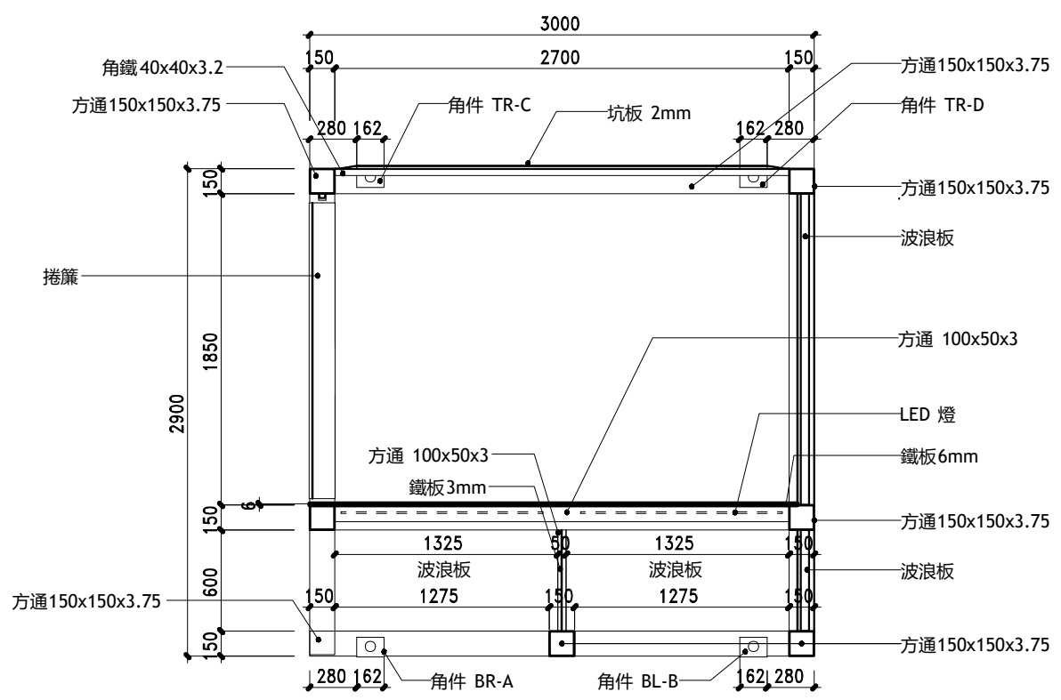
11-1F 剖面圖
